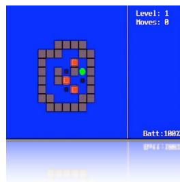
Sokoban
